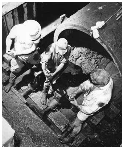
写真－1 手押しシップジャッキを用いた初期の押管作業（昭和27年頃）
