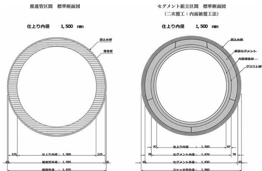
図-2 施工断面図（仕上り内径φ1,500mm）
