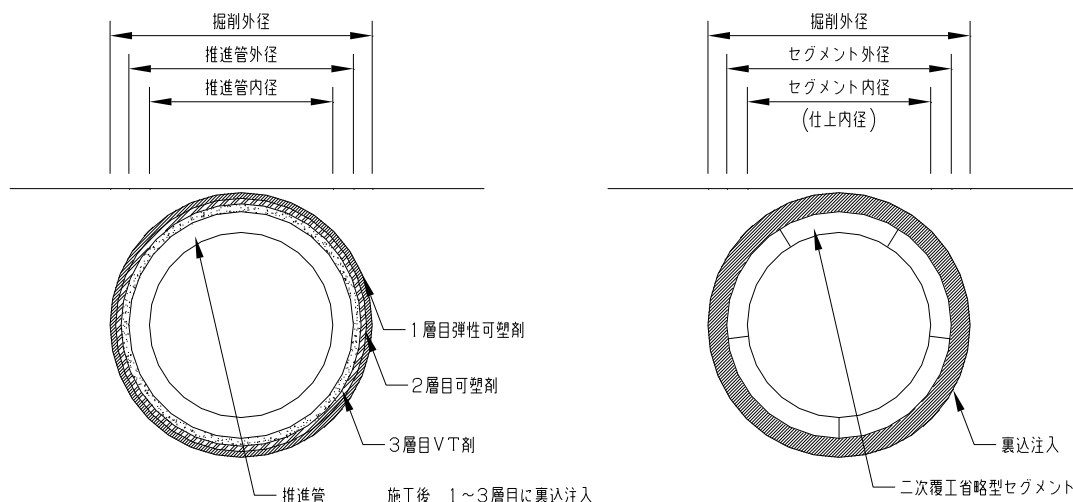
図-2 推進工法区間およびシールド工法区間標準断面図
