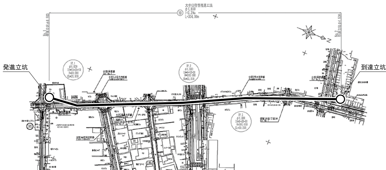
图-1 施工平面图
