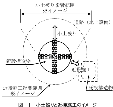
図ー1 小土被りと近接施工のイメージ
