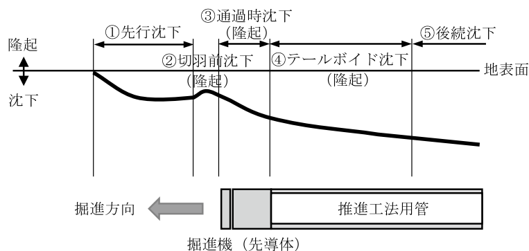
図ー2 掘進による経時変位イメージ
