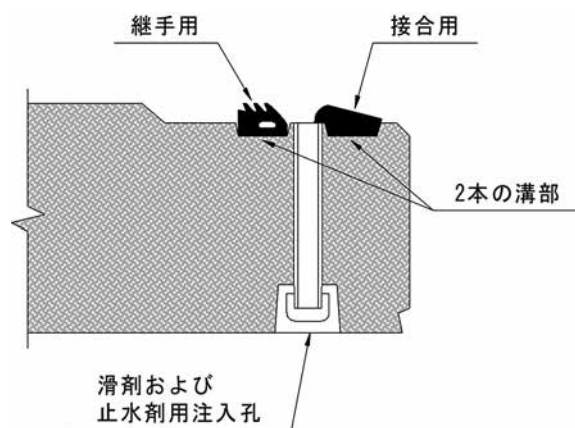
図-1 Wジョイント管の継手
