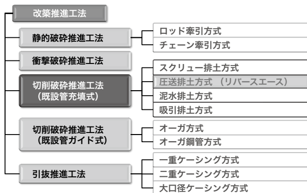
図-2 改築推進工法の分類（(公社)日本推進技術協会資料抜粋）
