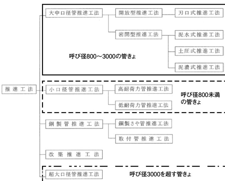
図-1 推進工法の分類
