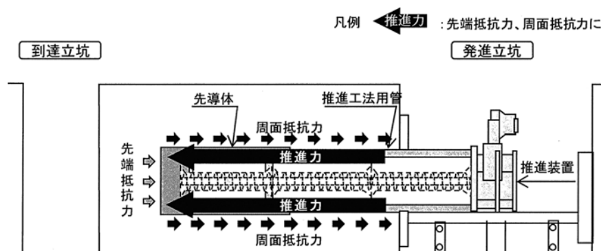
図-2 高耐荷力管推進工法（オーガ式）のイメージ 出典：推進工法体系Ⅰ 推進工法技術編2019年改訂版（本協会図書）
