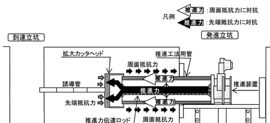
図-3 低耐荷力管推進工法（圧入式）のイメージ 出典：推進工法体系Ⅰ 推進工法技術編2019年改訂版（本協会図書）
