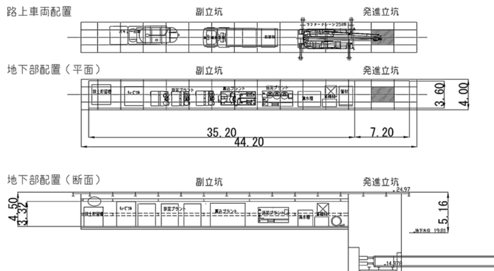
図－2 地下利用式プラント
