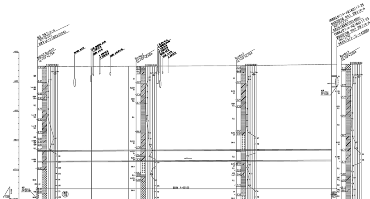
図-2 縦断面図
