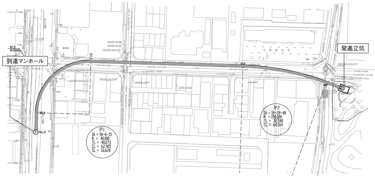
図-1 平面図
