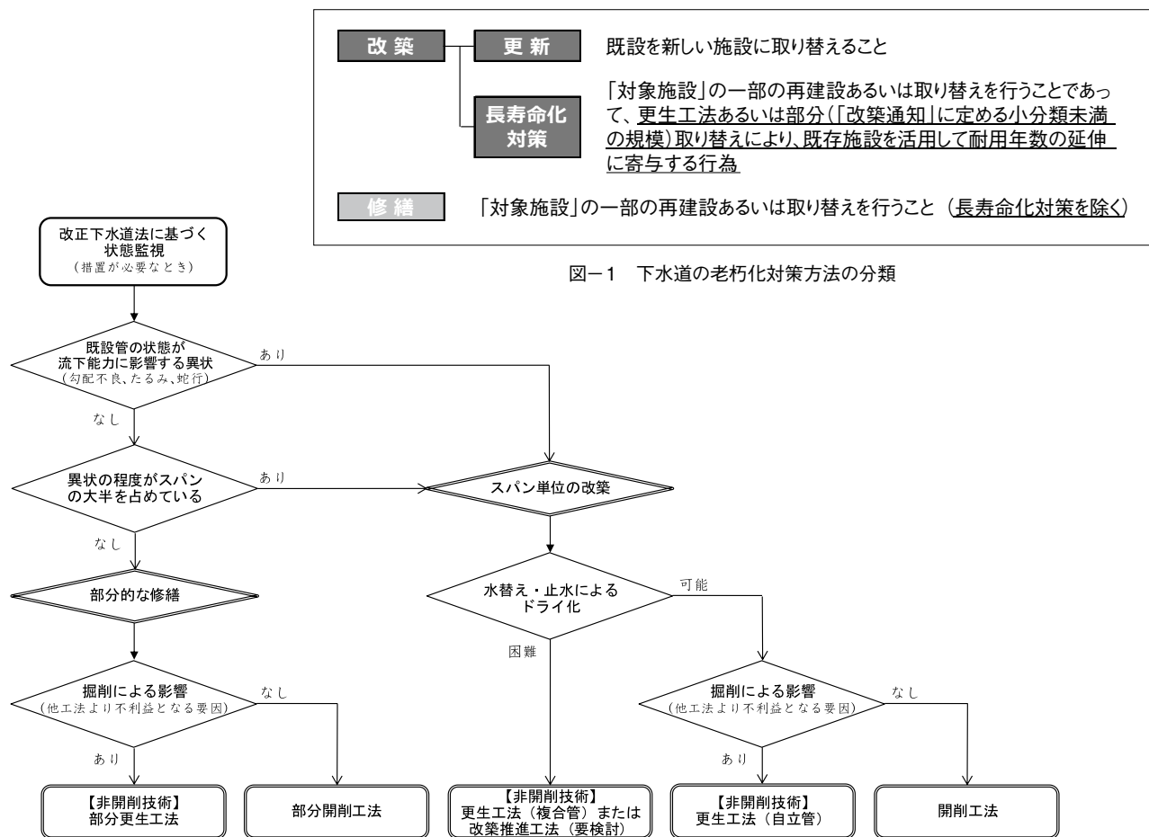
図－2 下水管きょの老朽化対策検討フロー
