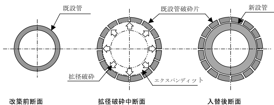
図-2 改築推進過程の管路断面図
