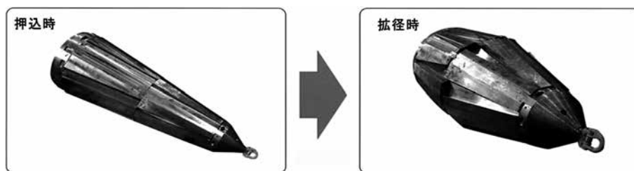
写真-1 エキスパンディットの可動状況
