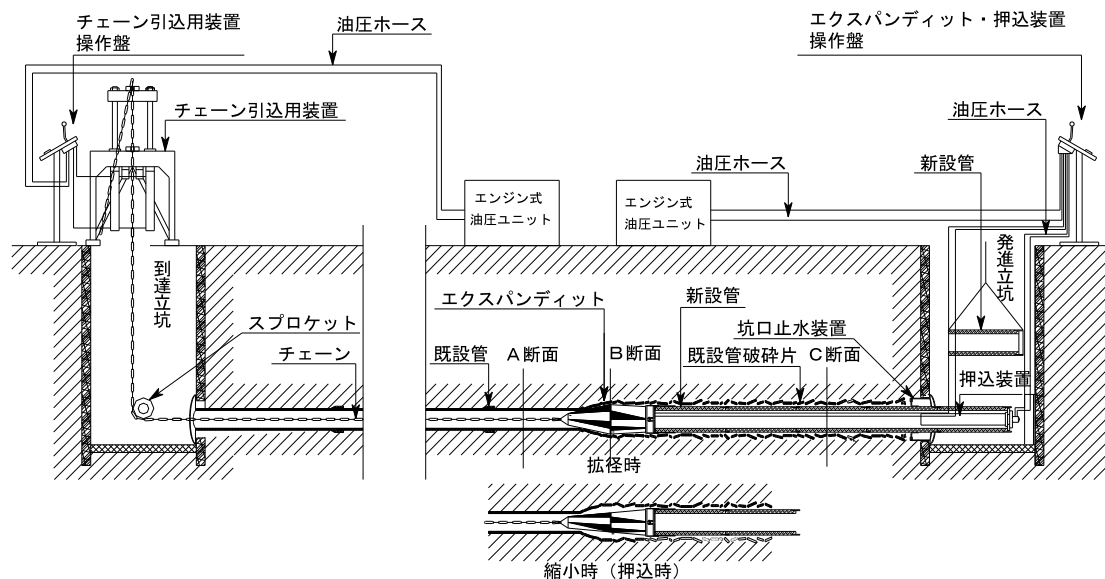
図-1 EXP工法の設備、施工概要
