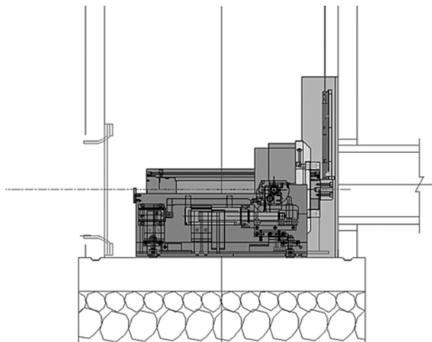
図-3 KRMジャッキ据付け断面図（1号マンホール）
